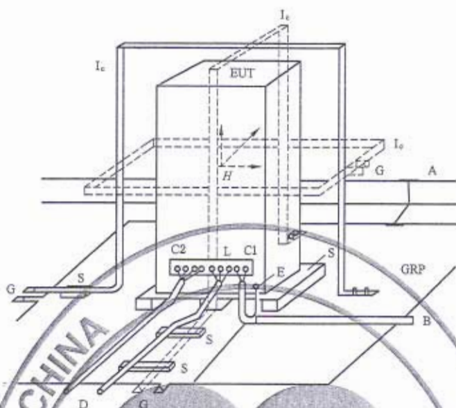
GRP—接地平面; C1—供电回路; A—安全接地; C2—信号回路; S—绝缘支座; L—通信线路; EUT—受试设备; E—至电源; Ic—感应线圈; D—至信号源, 模拟器; E—接地端子; G—至试验发生器
