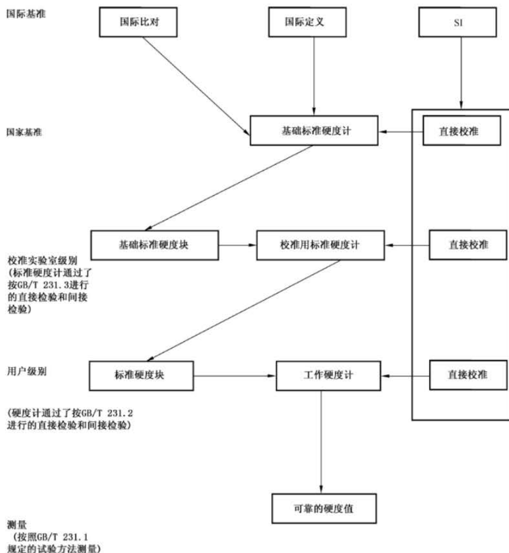
图 C.1 硬度标尺的定义和量值传递图
