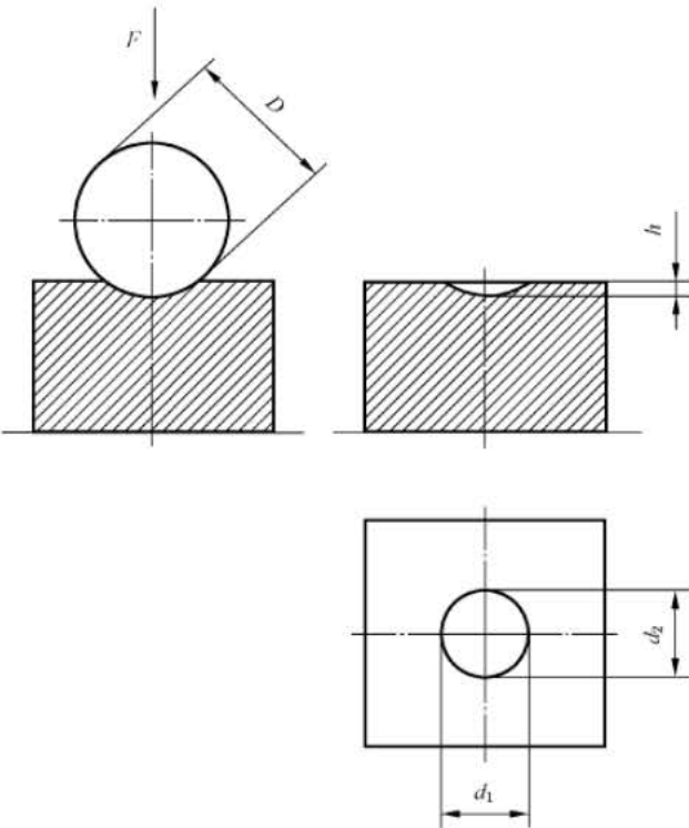
图 1 试验原理
