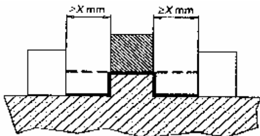
例 6 所测量的路径包含一条未粘合的接缝，该接缝的两侧各有一条宽度大于或等于 X 的沟槽。 电气间隙是“视线”的距离。 爬电距离是沿沟槽轮廓线伸展的通路。
