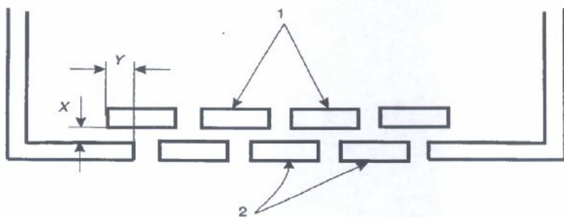
Y \geq 2X 但不小于 25 mm 1——挡板（可以位于外壳底部的下面）； 2——外壳底部
