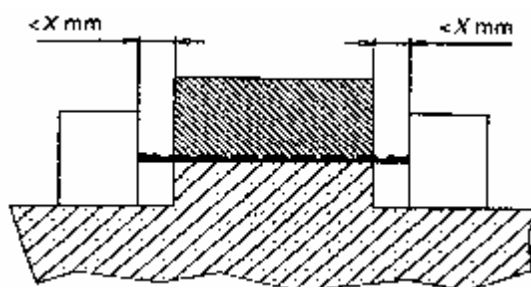
例 5 所测量的路径包含一条未粘合的接缝，该接缝的两侧各有一条宽度小于 X 的沟槽。 爬电距离和电气间隙是如图所示的“视线”的距离。
