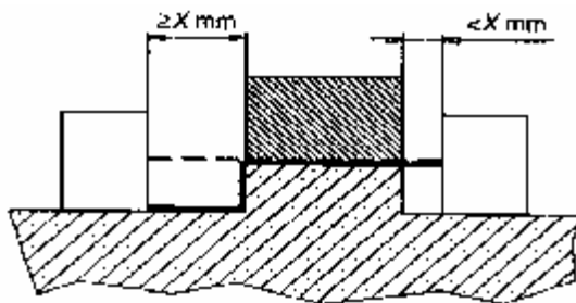
例 7 所测量的路径包含一条未粘合的接缝，该接缝的一侧有一条宽度小于 X 的沟槽，另一侧有一条宽度等于或大于 X 的沟槽。 爬电距离和电气间隙如图所示。
