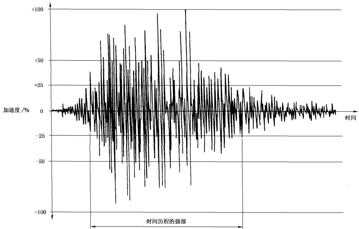
图 4 典型时间历程
