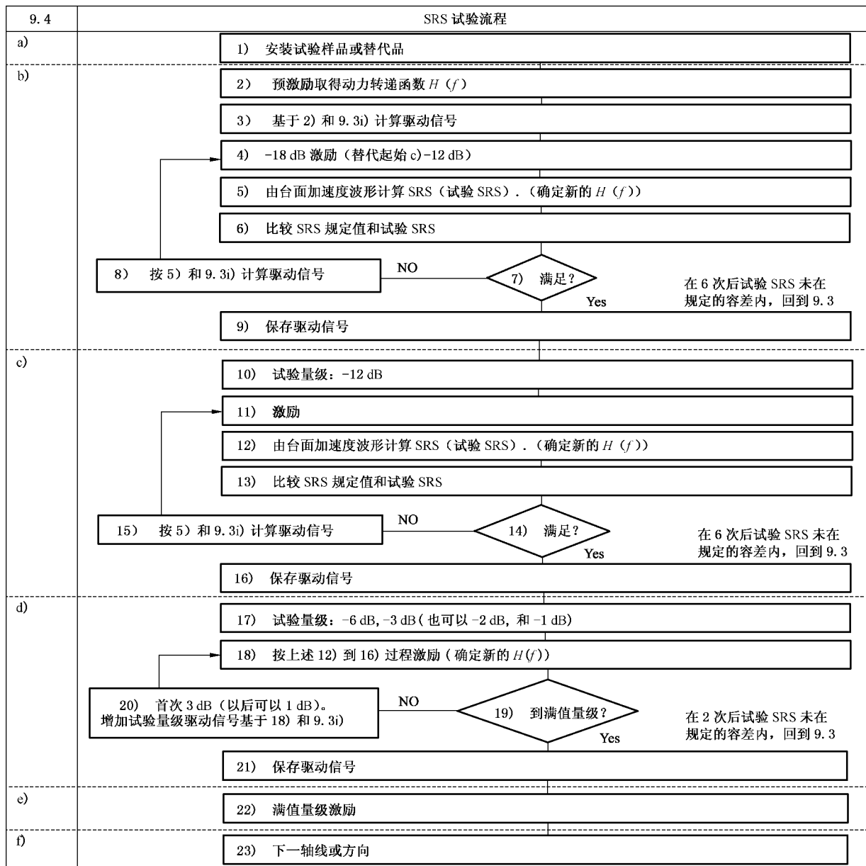
图 5 合成时间历程试验的流程图(9.4)
