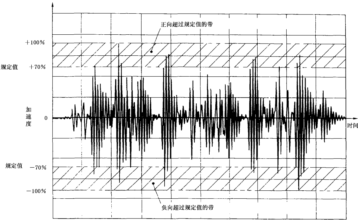
图 1 典型的由特定时间历程激励的响应示例(规定阈值 70%)
