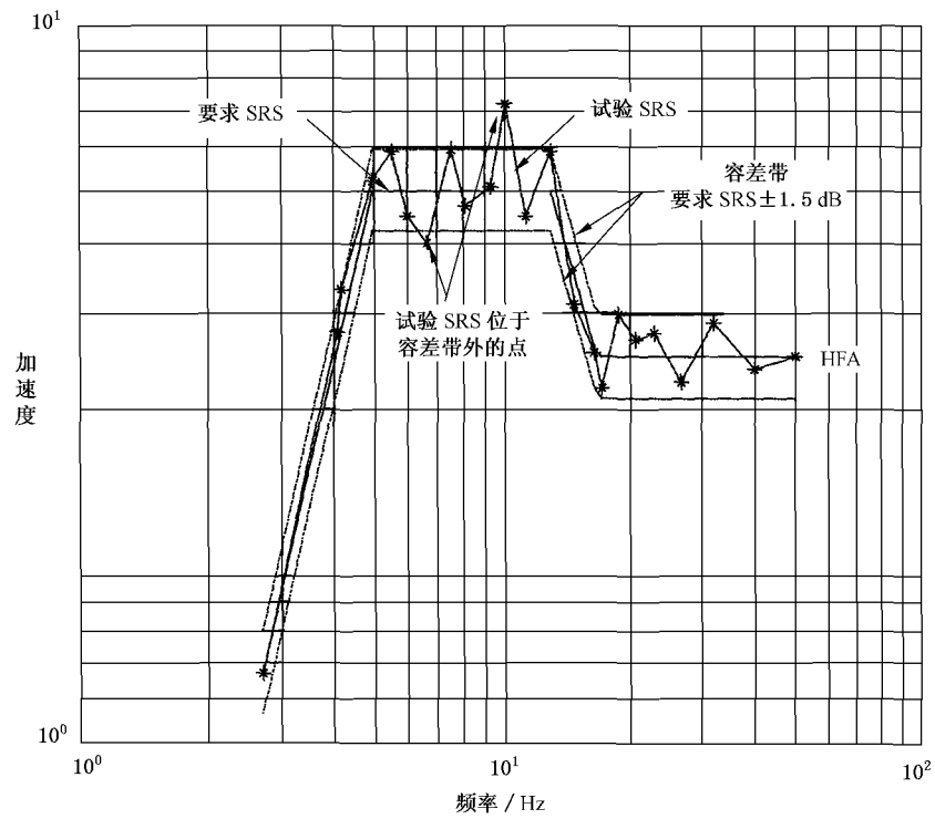
图 3 要求响应谱的典型对数图
