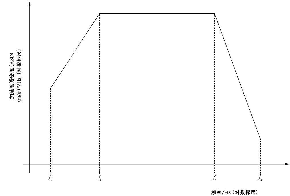
图 A.2 固定安装谱线——频率/振幅断点
