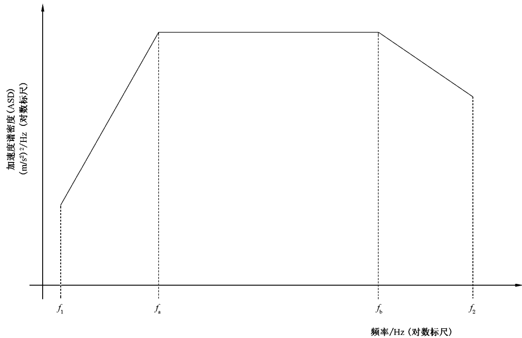
图 A.3 轮式车设备——频率/振幅断点
